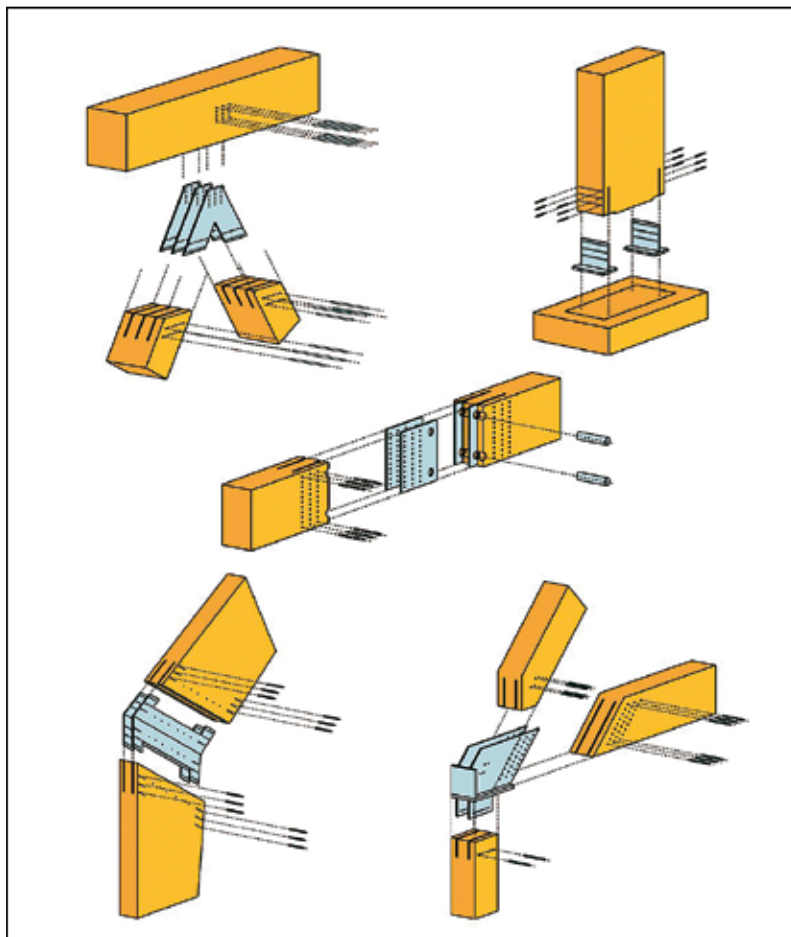
Joonis 1. Mõningaid variante sissefreesitud plaatide ja puurkruidudega liidetest. JOONIS: SFS INTEC
